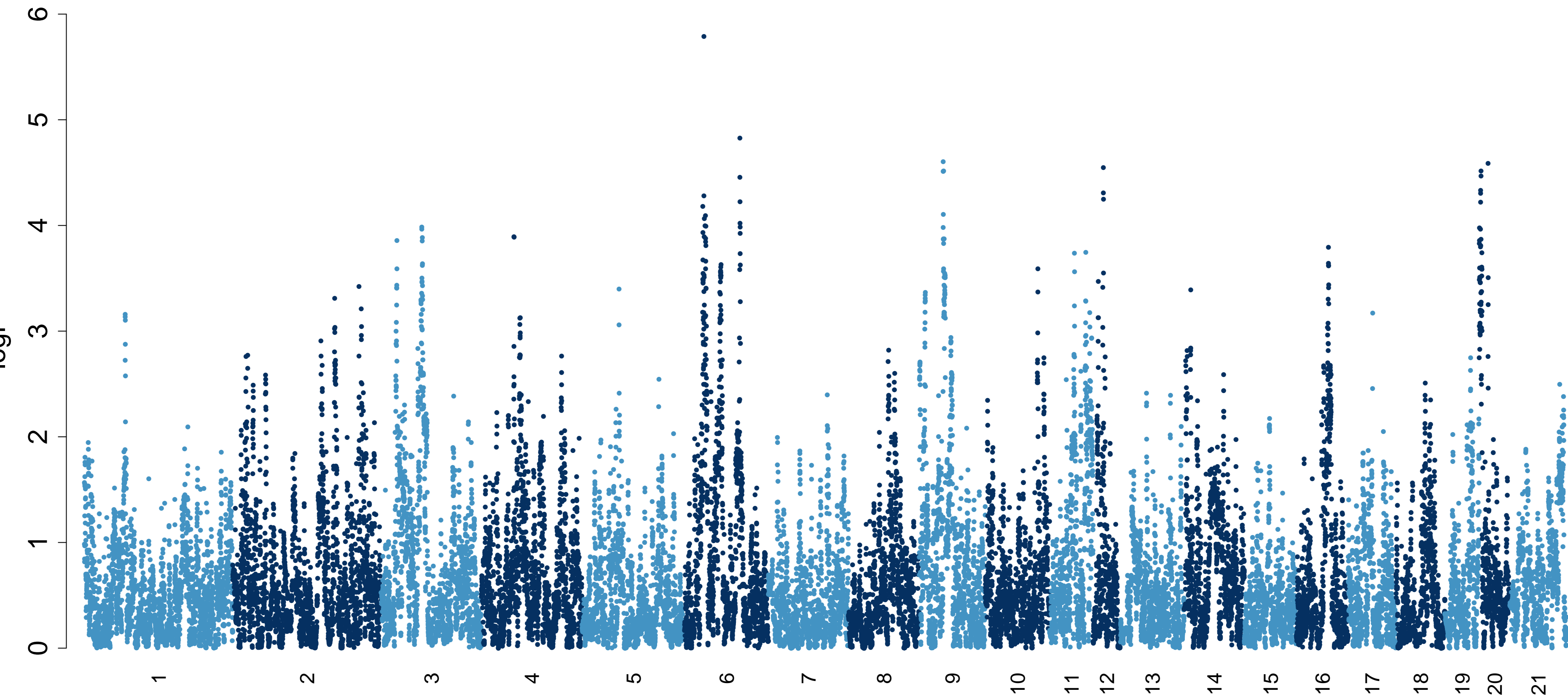
Bone_femur_midshaft_CRT_DEN
