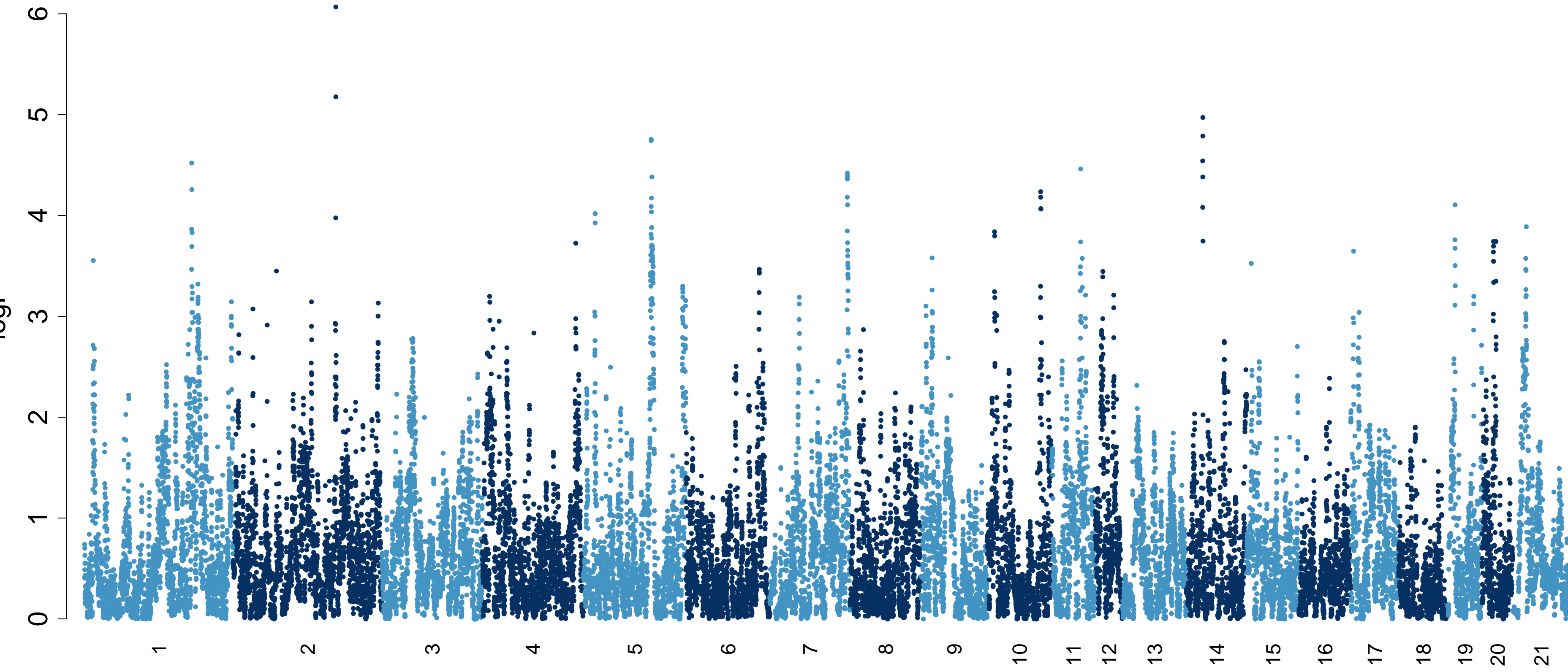
Bone_lumbar_BMD
