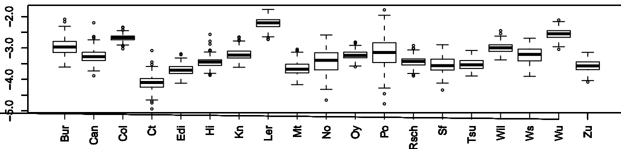
basal.given.days.to.bolt MN1_112907 chr1 20806858
