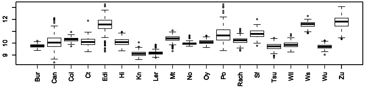
bolt.to.flower MN1_112907 chr5 658143
