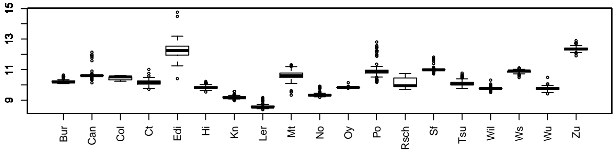
bolt.to.flower MASC03771 chr5 3281888
