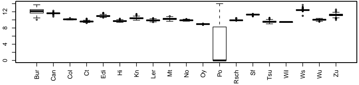
bolt.to.flower MN1_129776 chr4 125591 4
