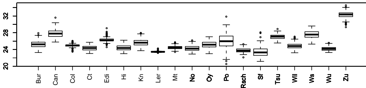
days.to.bolt MN1_112907 chr4 7177635
