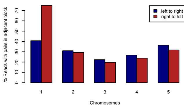
MAGIC.446 – DENSE.BPS
