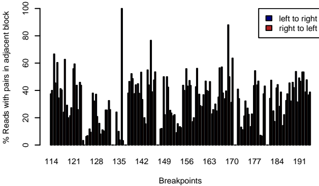
MAGIC.105 – DENSE.BPS
