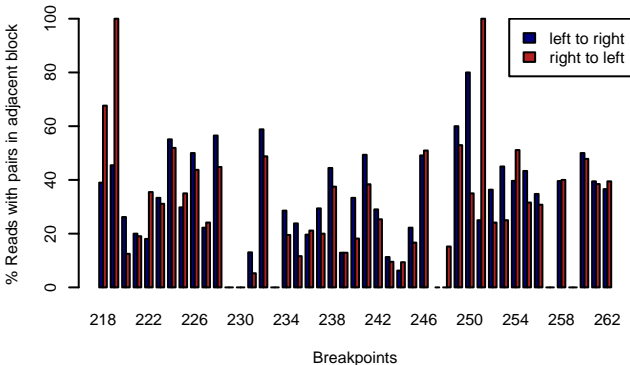
MAGIC.446 – DENSE.BPS
