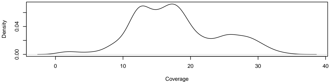
MAGIC.175 5 13948032 13948034
