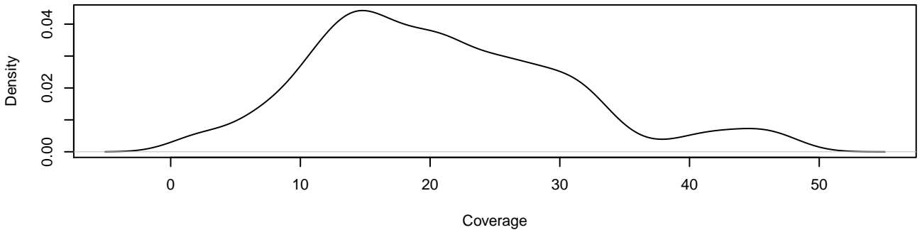
MAGIC.175 3 23019788 23019789
