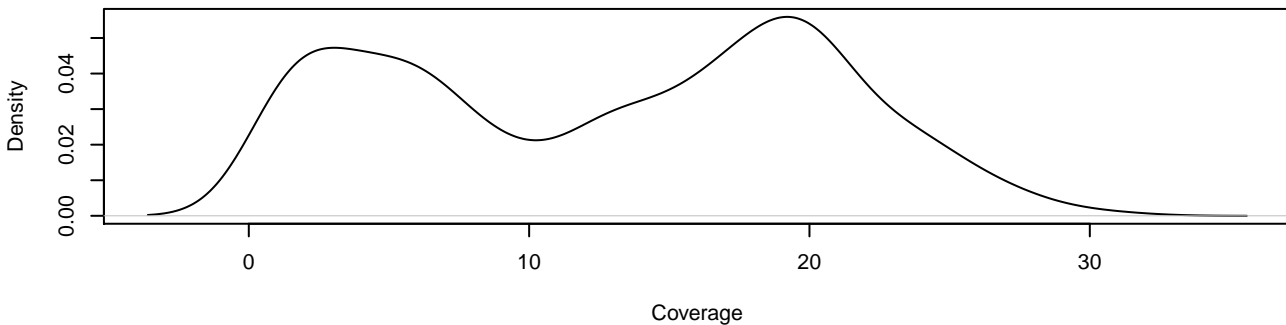
MAGIC.175 5 5647354 5647357
