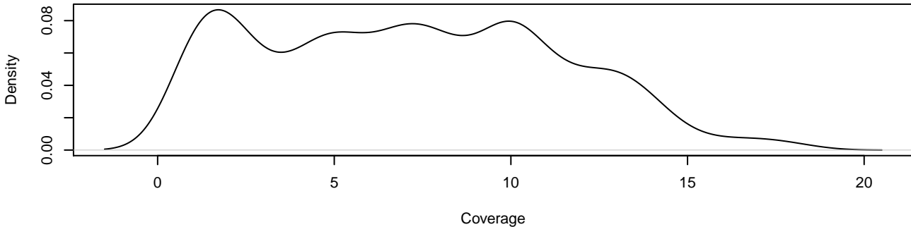
MAGIC.175 5 10064972 10064987
