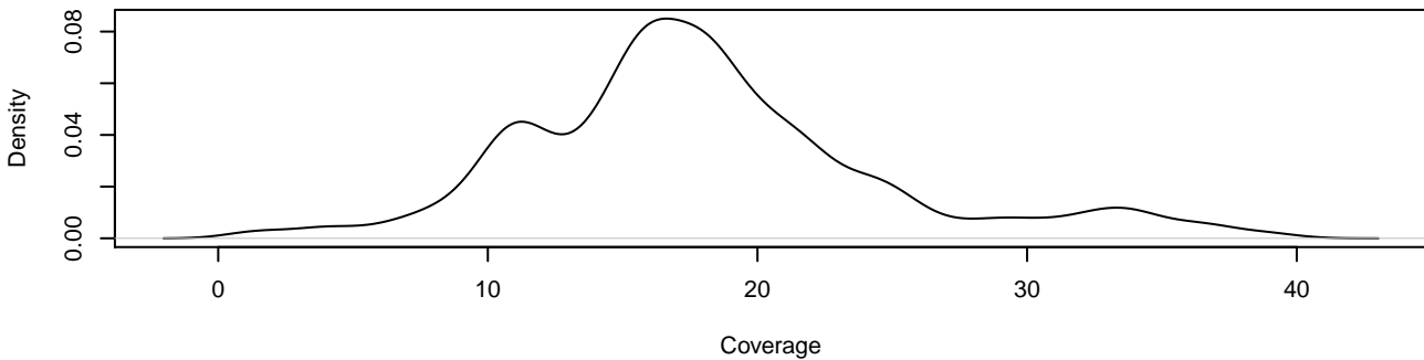
MAGIC.175 4 9583248 9583261
