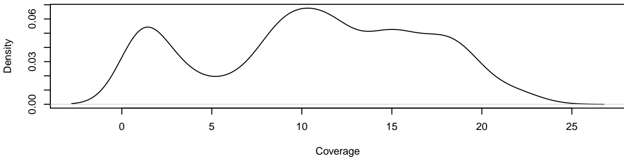
MAGIC.446 4 1027588 1027593
