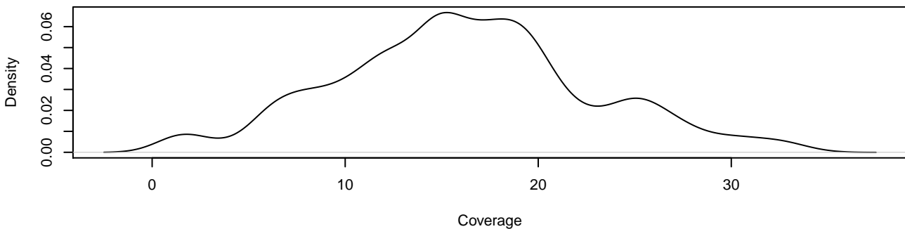
MAGIC.446 1 9444643 9444646
