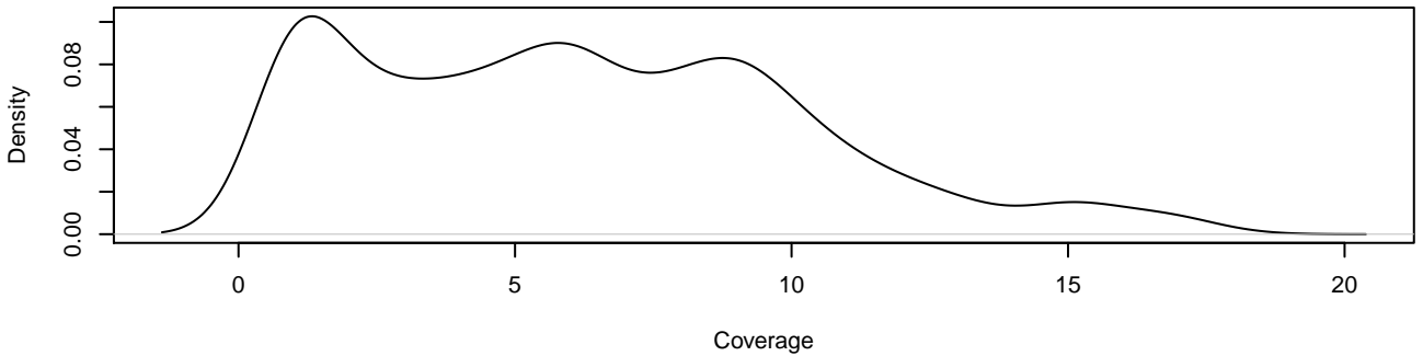
MAGIC.446 4 1909491 1909539
