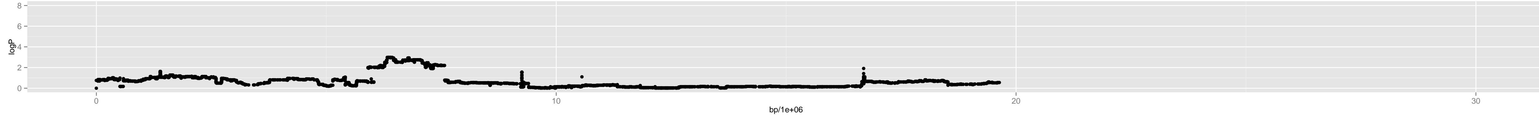
Chromosome 2 – 1_rschr.4_15504886_5_5
