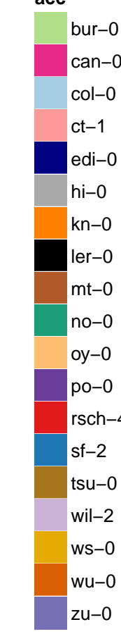
acc
