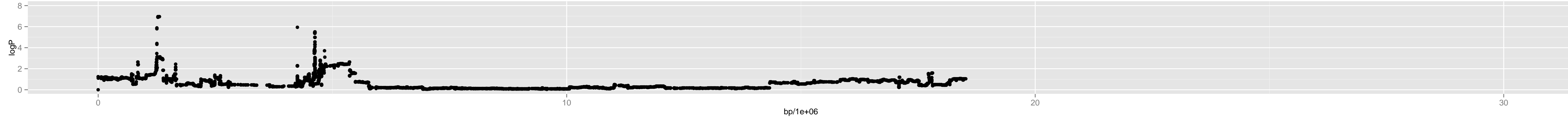
Chromosome 4 – 5_bur.0_20299561_11_6
