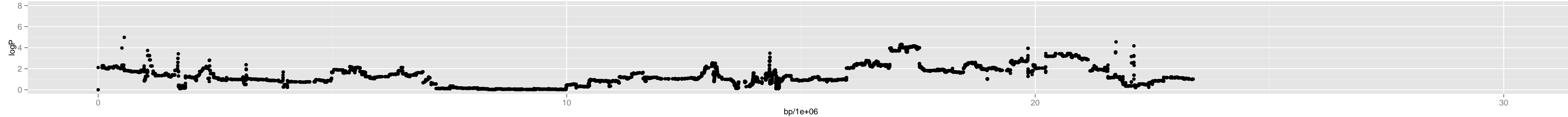
Chromosome 3 – 5_bur.0_20299561_11_6
