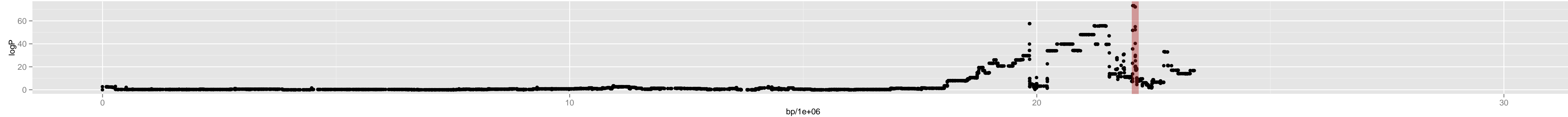
Chromosome 3 – 3_bur.0_22107508_9_9
