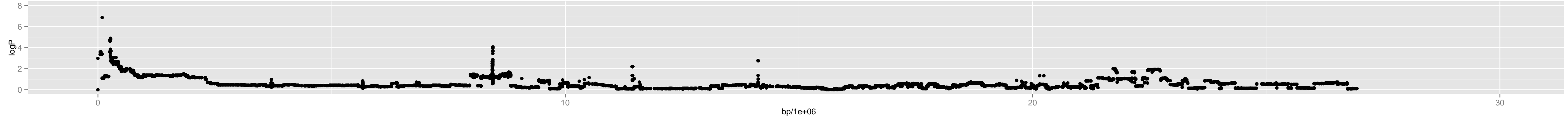
Chromosome 5 – 3_rsch.4_13957881_6_5
