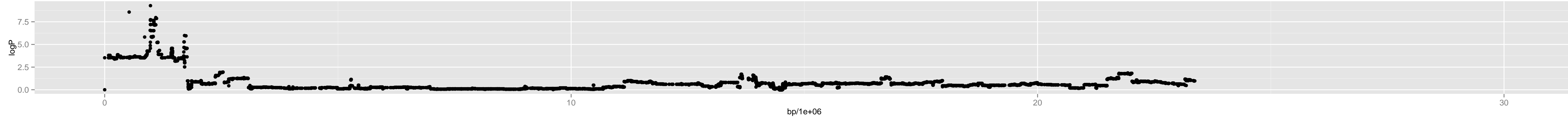
Chromosome 3 – 5_zu.0_14050321_9_3
