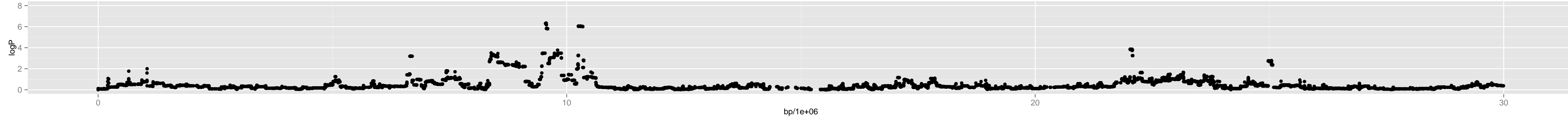
Chromosome 1 – 3_wil.2_14444678_20_6
