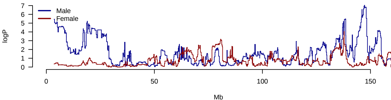
AUC.IRI.AUC.G Chromosome 3
