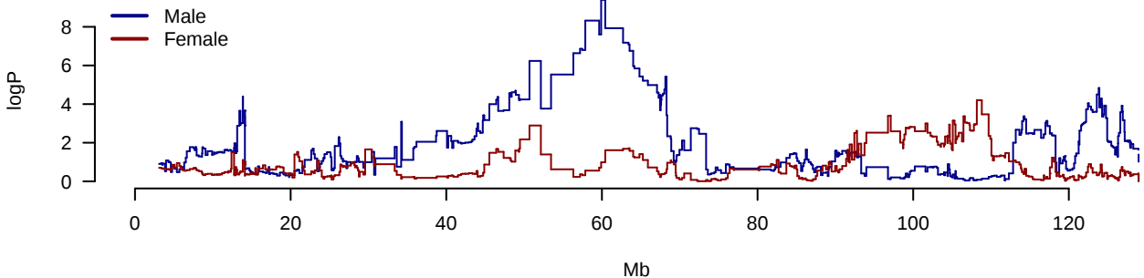
AUC.IRI.AUC.G Chromosome 11
