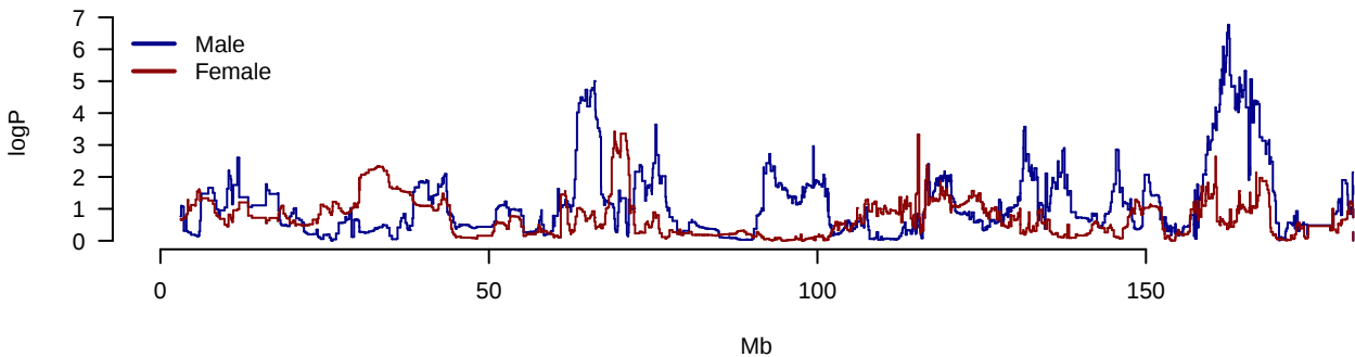
AUC.IRI.AUC.G Chromosome 2
