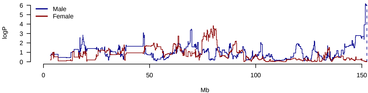
AUC.IRI.AUC.G Chromosome 7
