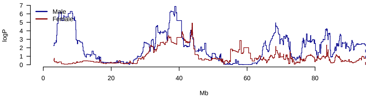
AUC.IRI.AUC.G Chromosome 17
