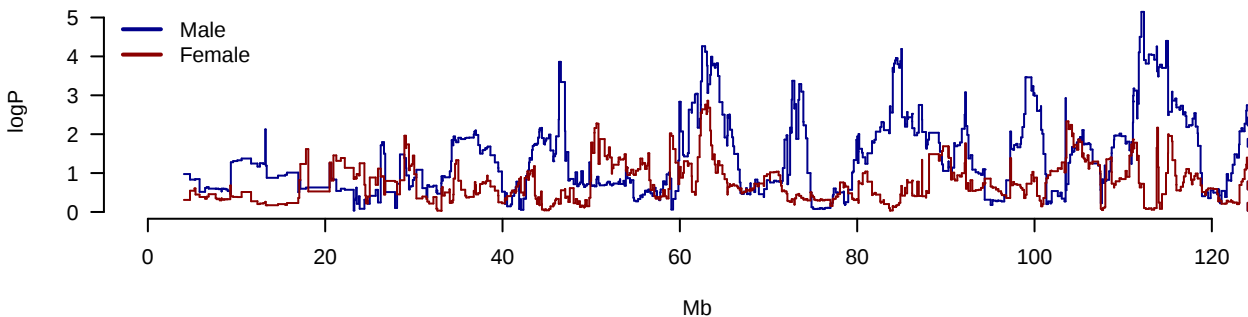
AUC.IRI.AUC.G Chromosome 9
