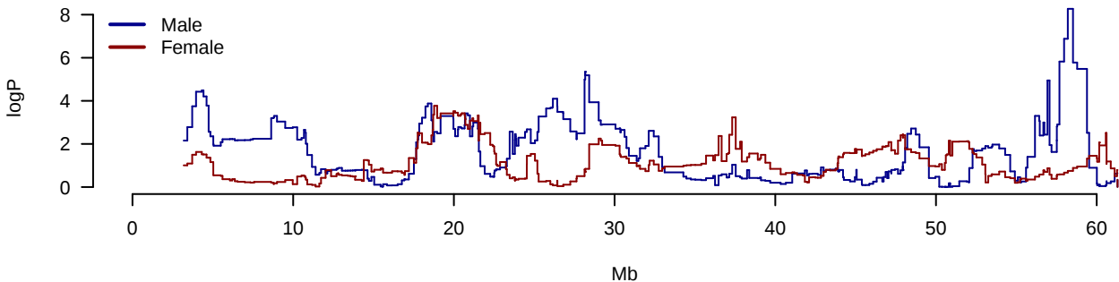
AUC.IRI.AUC.G Chromosome 19
