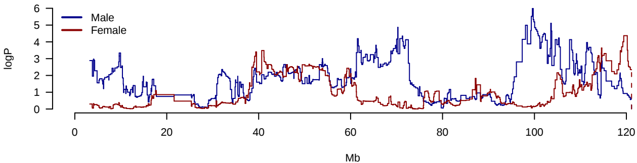
AUC.IRI.AUC.G Chromosome 12
