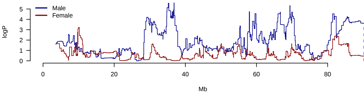
AUC.IRI.AUC.G Chromosome 18
