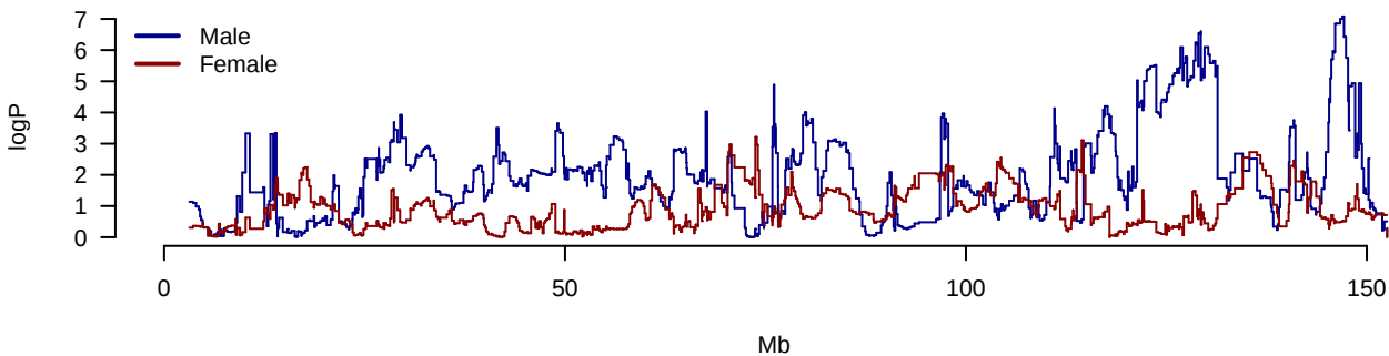
AUC.IRI.AUC.G Chromosome 5
