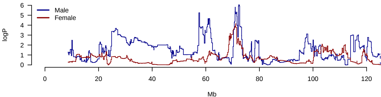
AUC.IRI.AUC.G Chromosome 14
