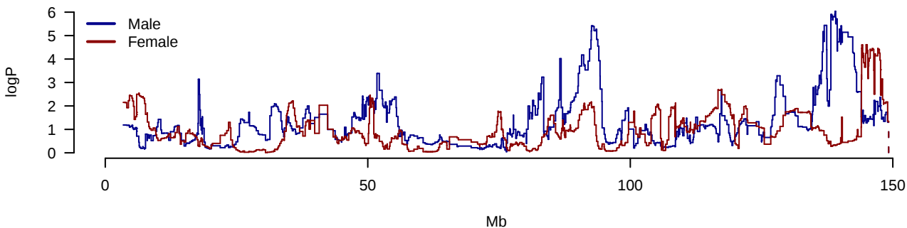
AUC.IRI.AUC.G Chromosome 6
