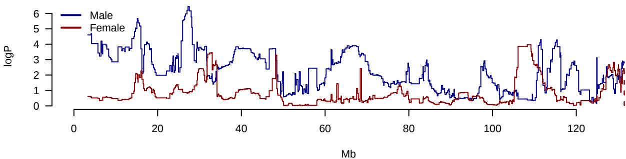
AUC.IRI.AUC.G Chromosome 8
