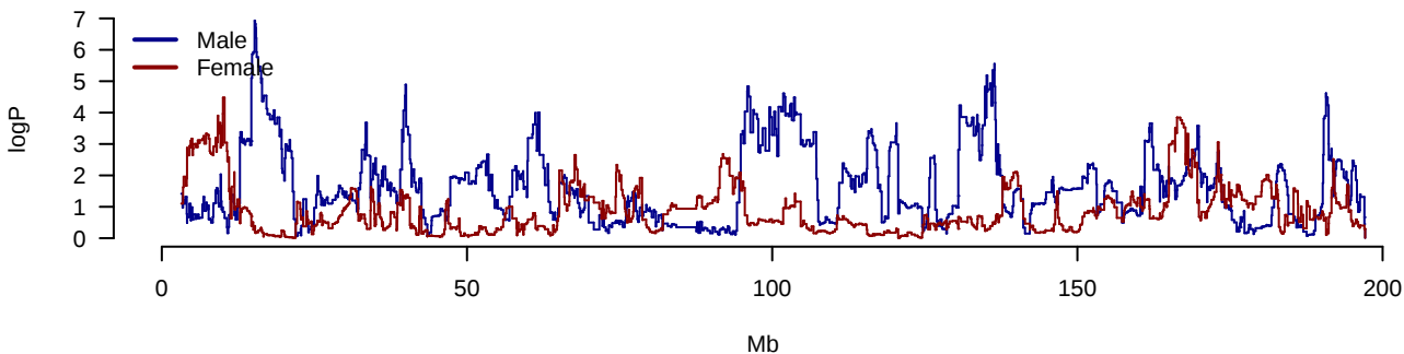
AUC.IRI.AUC.G Chromosome 1
