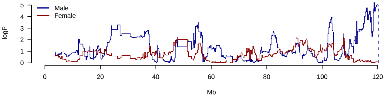
AUC.IRI.AUC.G Chromosome 14
