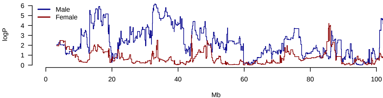
AUC.IRI.AUC.G Chromosome 15
