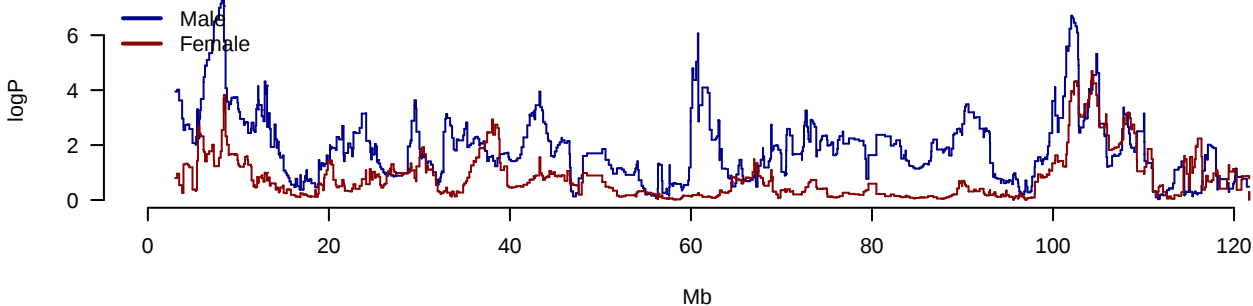
AUC.IRI.AUC.G Chromosome 12
