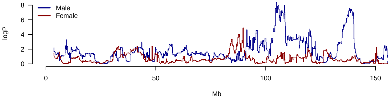
AUC.IRI.AUC.G Chromosome 5
