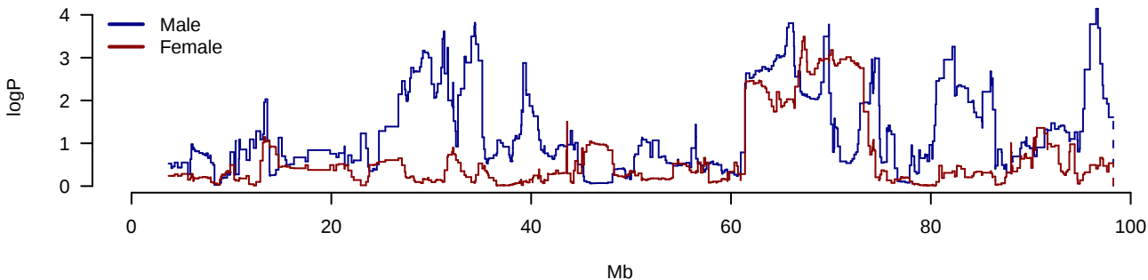
AUC.IRI.AUC.G Chromosome 16
