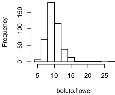
bolt.to.flower
