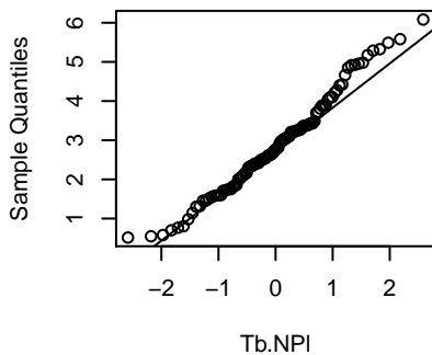
Tb.NPI
