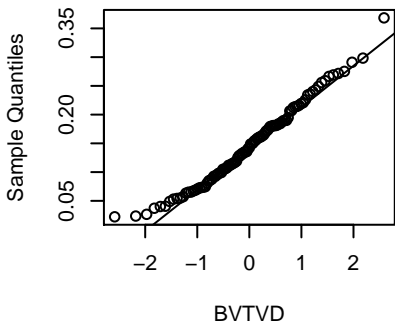
BVTVD
