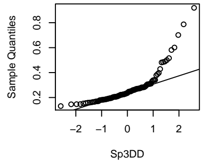
Sp3DD
