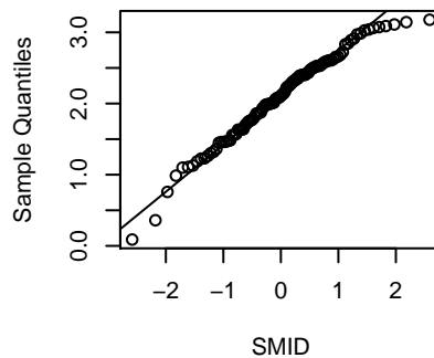
SMID
