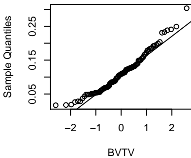
BTV
