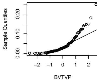
BVTVP
