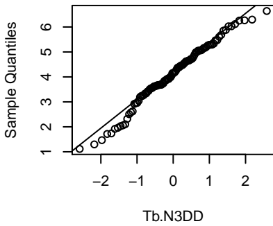
Tb.N3DD
