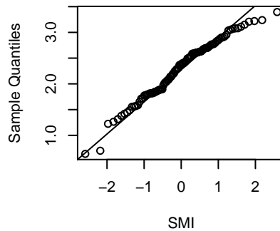
SMI
