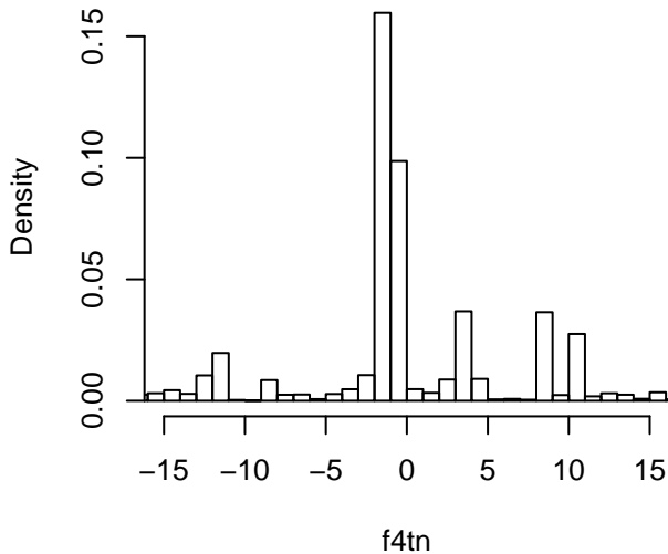
Tb.N
