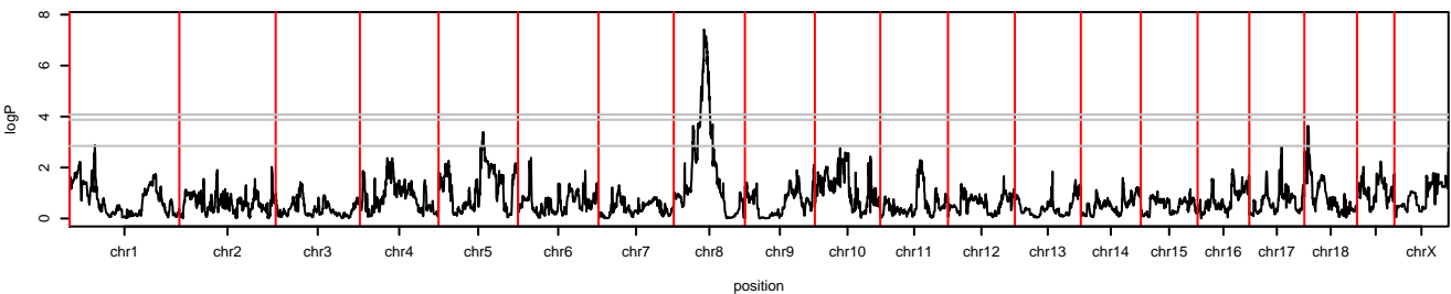
Tb.Th.met
