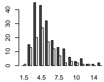
AUC
