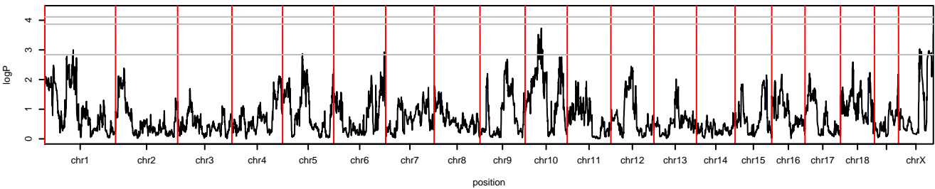
SMID
