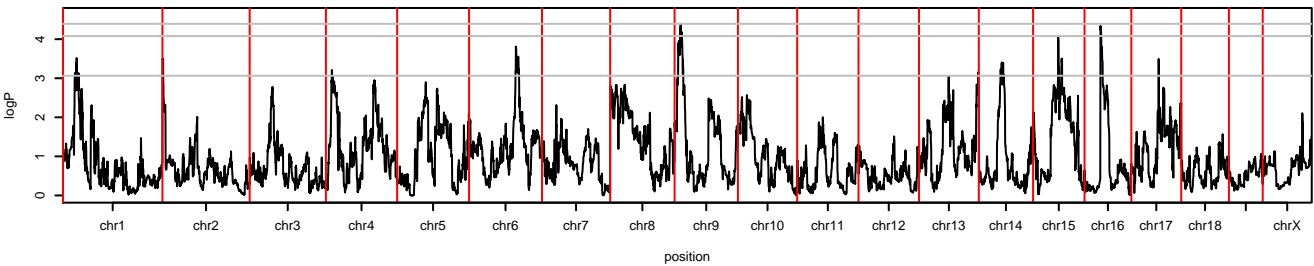
Tb.ThD
