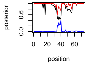
IL-313 Chr chr14
