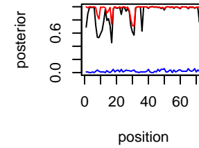
IL-636 Chr chr14
