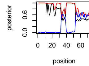
IL-507 Chr chr14
