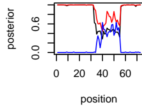
IL-530 Chr chr14
