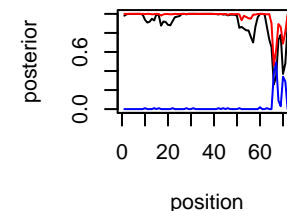
IL-549 Chr chr14
