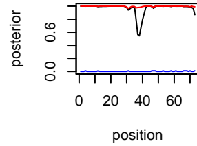
IL-18 Chr chr14
