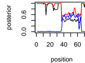
IL-177 Chr chr14
