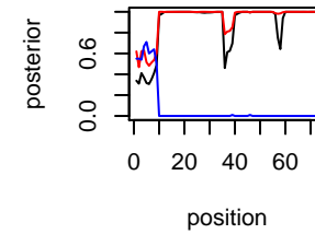
IL-640 Chr chr14
