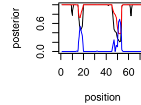
IL-599 Chr chr14
