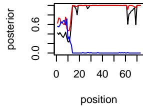
IL-312 Chr chr14
