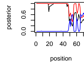
IL-39 Chr chr14
