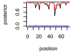
IL-134 Chr chr14
