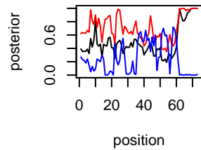
IL-104 Chr chr14
