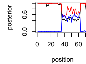
IL-217 Chr chr14
