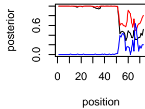
IL-717 Chr chr14
