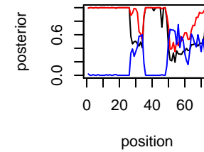
IL-627 Chr chr14
