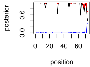
IL-19 Chr chr14
