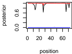
IL-111 Chr chr14
