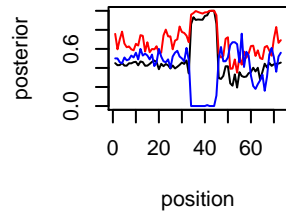
IL-127 Chr chr14
