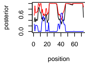
IL-196 Chr chr14
