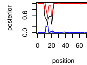
IL-604 Chr chr14
