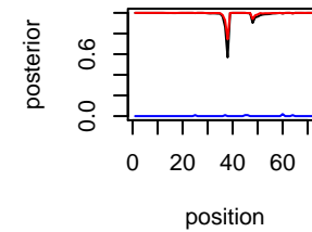
IL-634 Chr chr14
