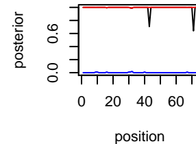
IL-55 Chr chr14
