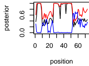
IL-290 Chr chr14
