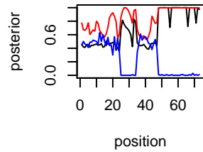
IL-188 Chr chr14
