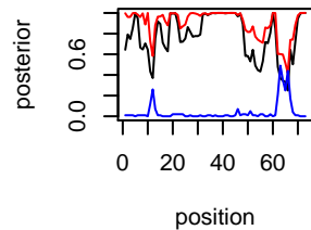
IL-317 Chr chr14
