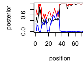
IL-547 Chr chr14
