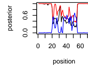
IL-699 Chr chr14
