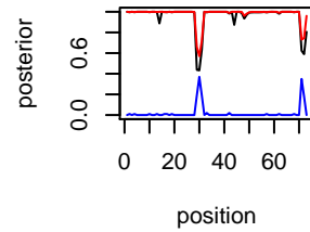
IL-15 Chr chr14
