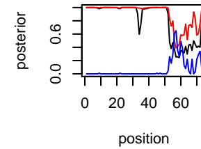
IL-521 Chr chr14
