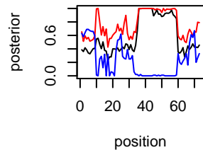
IL-294 Chr chr14
