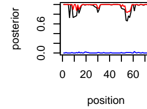
IL-511 Chr chr14
