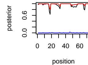
IL-817 Chr chr14
