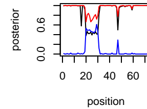
IL-517 Chr chr14
