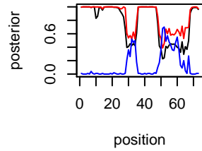
IL-287 Chr chr14
