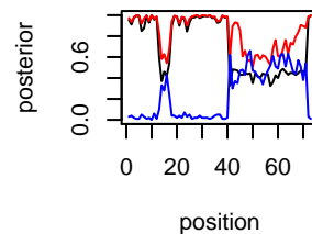
IL-619 Chr chr14
